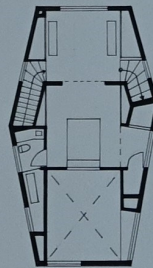
GRUNDRISS 1.OG
