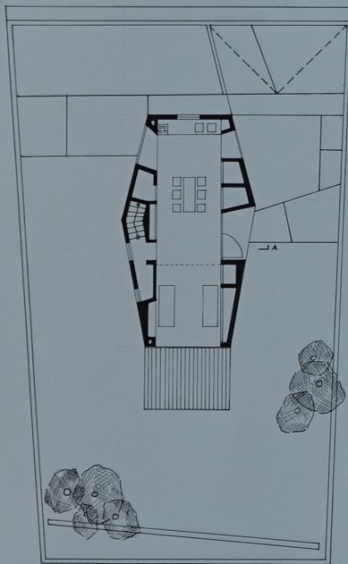
GRUNDRISS EG
