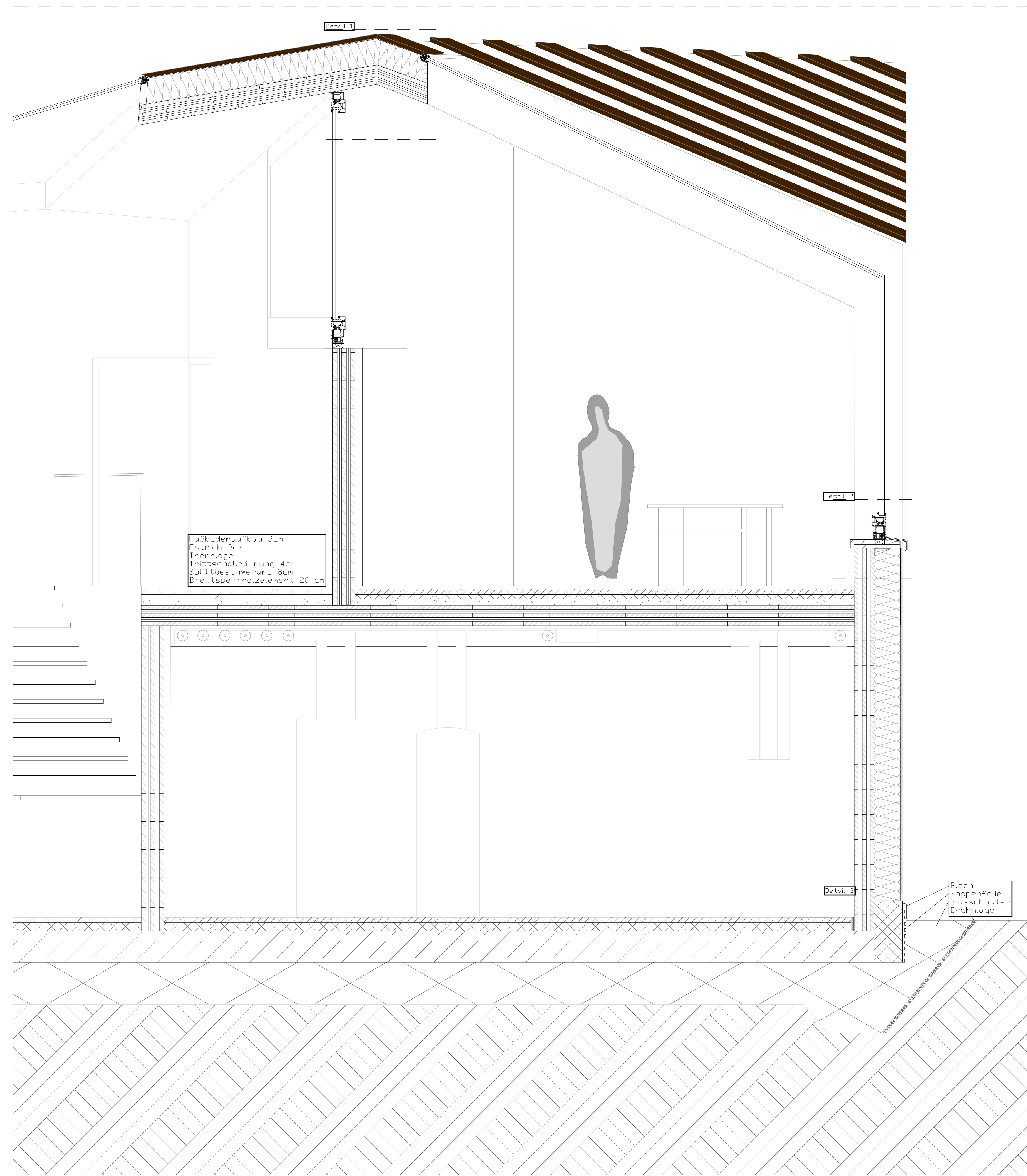
teilschnitt, 1:20
