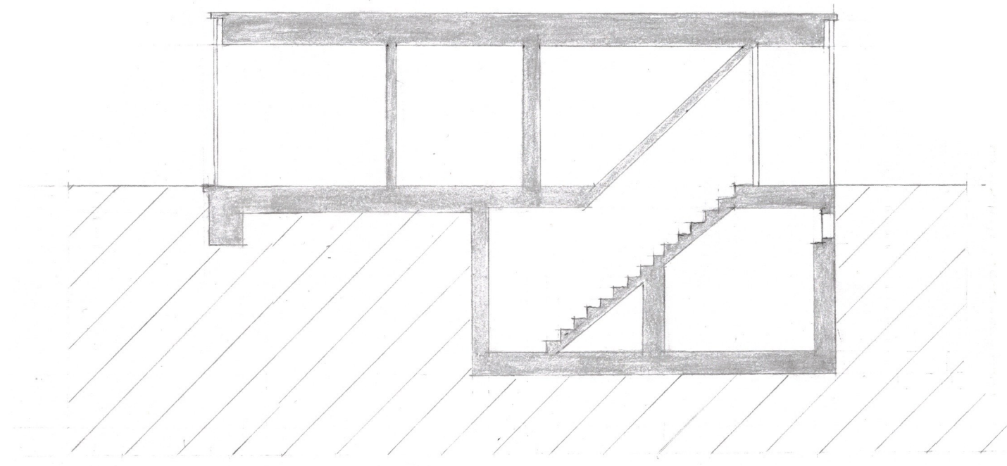
SCHNITT QUER
