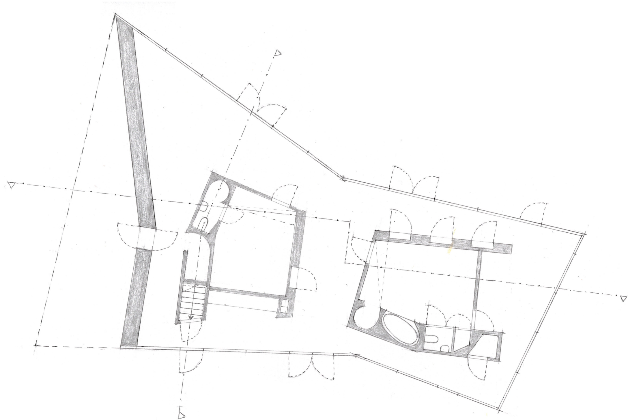
GRUNDRISS ERDGESCHOSS
