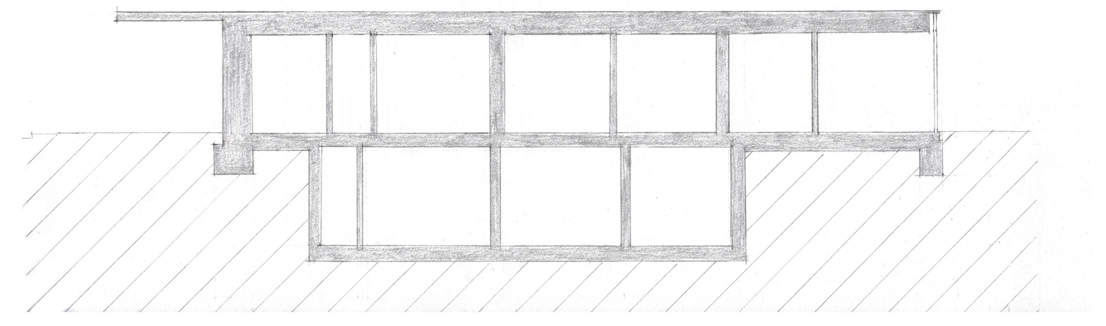
SCHNITT LÄNGS
