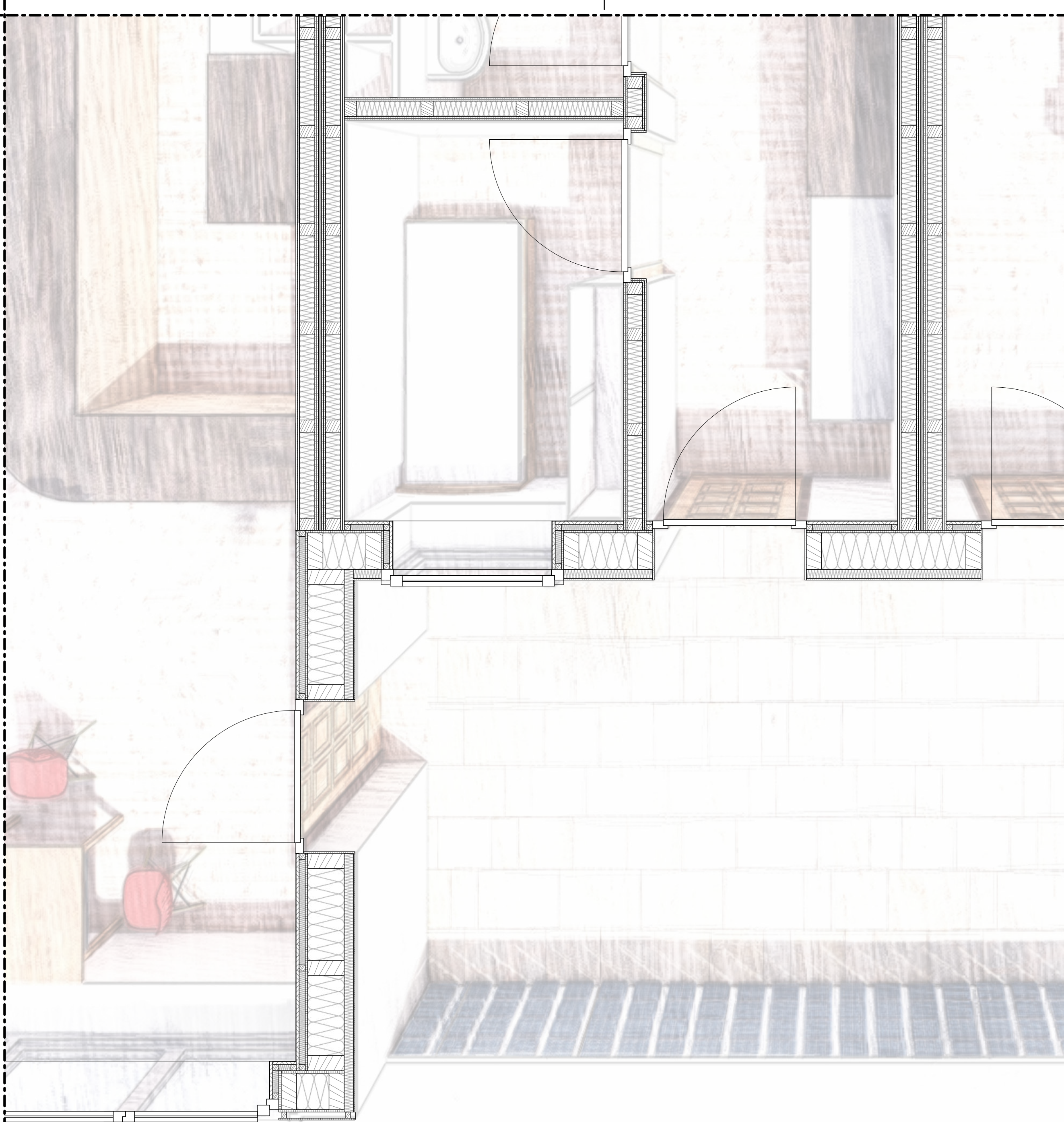
Grundrissausschnitt M 1:20
