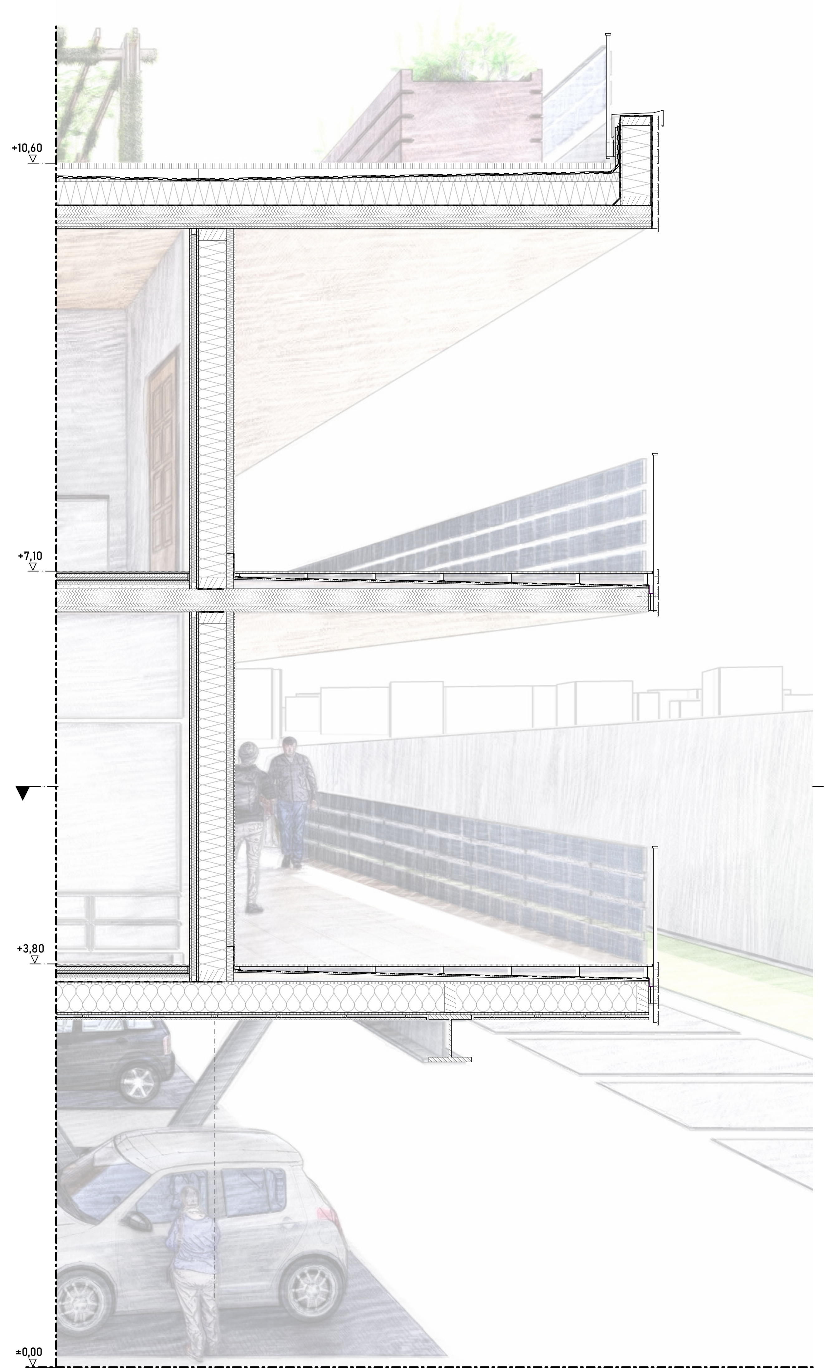
Fassadenschnitt M 1:20
