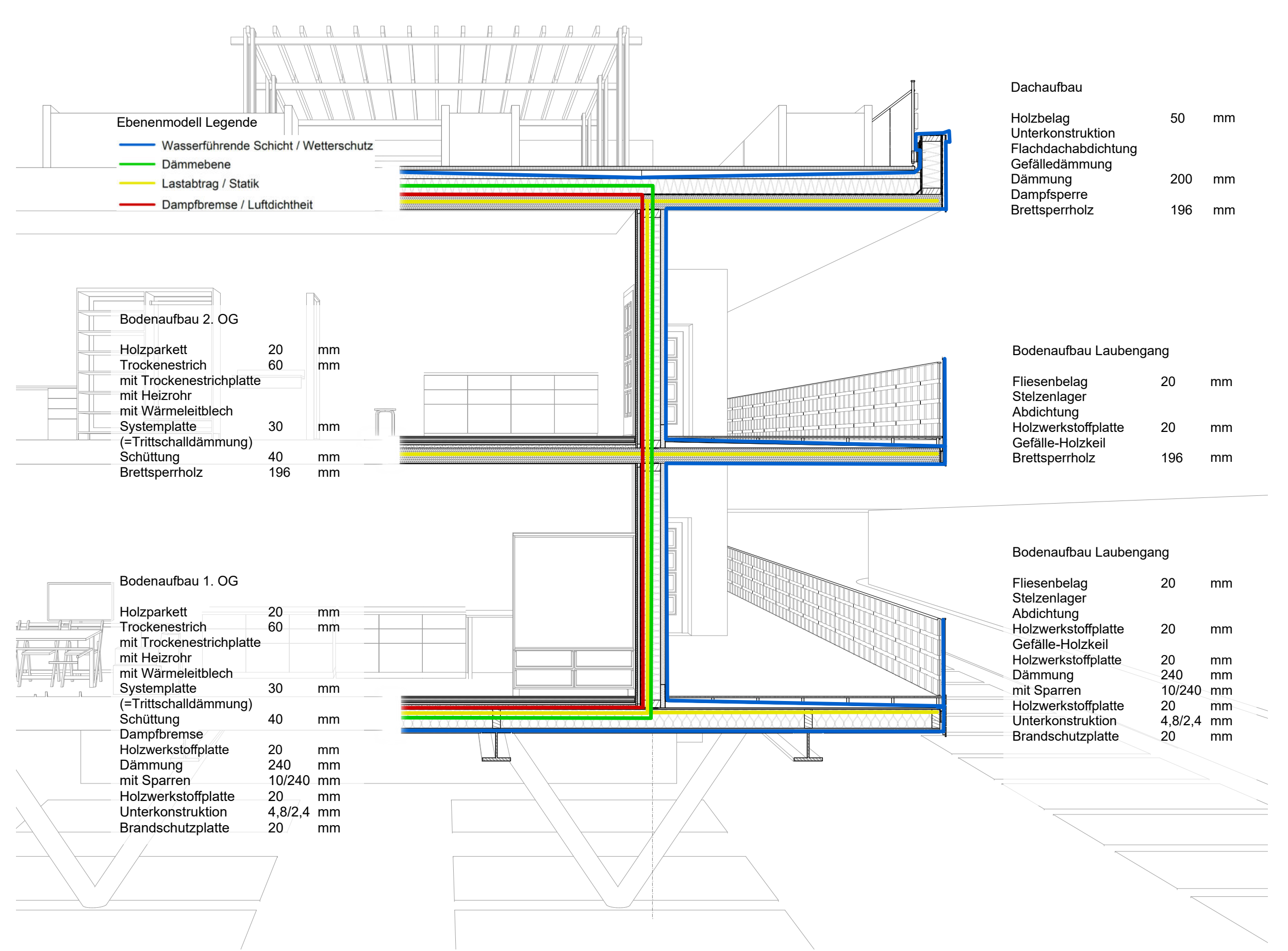
Ebenenmodell und Bodenaufbauten M1:50
