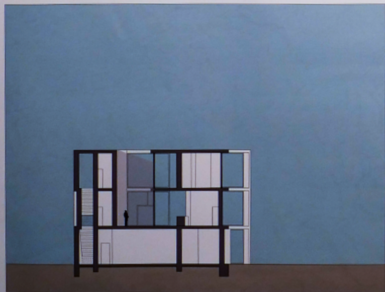
SCHNITT S1
