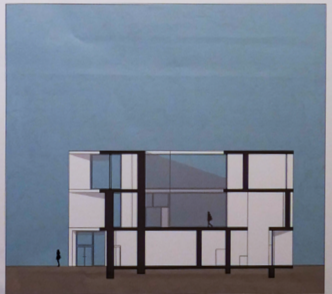
SCHNITT S2
