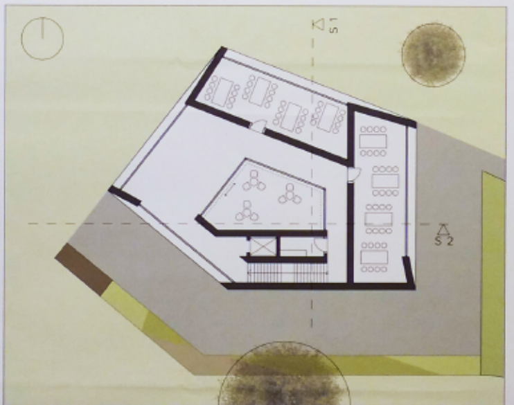
GRUNDRISS EG M 1:100
