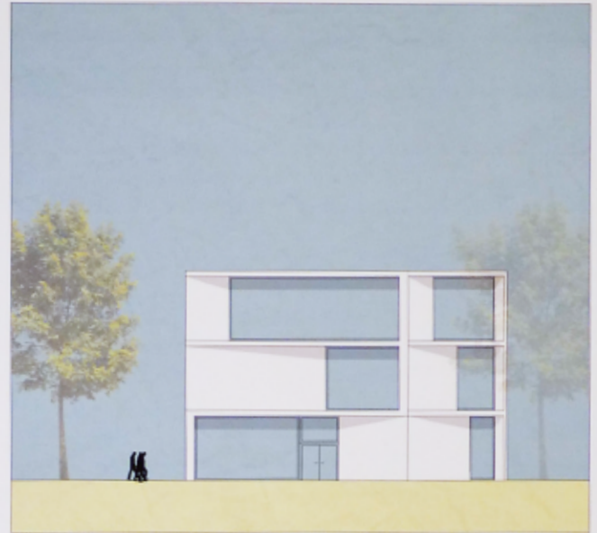
ANSICHT OST M1:100
