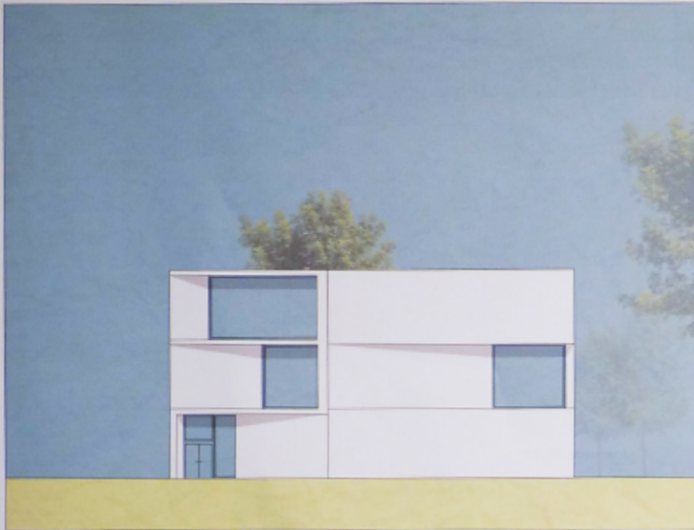
ANSICHT SÜD M1:100
